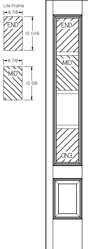
8 x 47 4 - Lite
