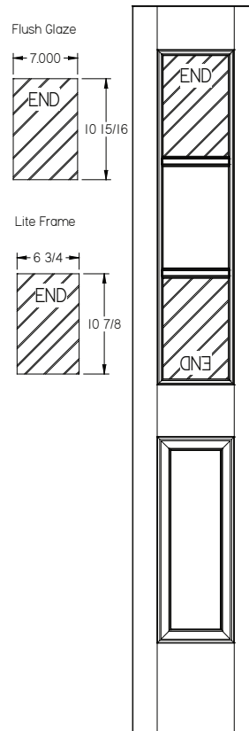
8 x 36 3 - Lite
